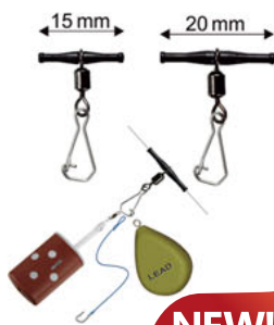
AS-721-15/AS-721-20 Stonfo, przelotowy łącznik do zestawów gruntowych.
