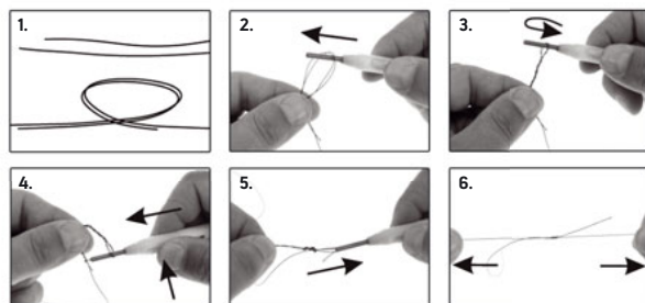
BEZPIECZNY WĘZEŁ ŁĄCZĄCY ŻYŁKĘ Z PLECIONKĄ
